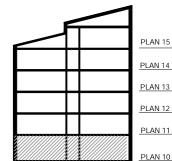
PRINCIPSEKTION A-A
